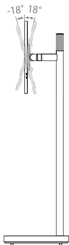
チルト角度 \pm 18.0^\circ ( \pm 2.0^\circ )
